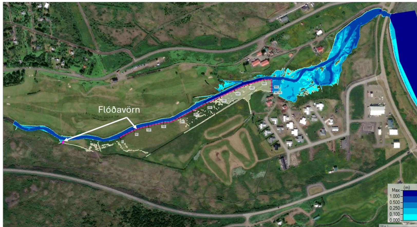
Mynd 5. Dýpi vatns við hönnunarflóð, 12 \text{ m}^3/\text{s} , með flóðavörn. Flóðavörnin er sýnd með bleikum lit á mynd. Útbreiðslu án flóðavarnar fyrir sama flóð er sýnd með gráum fláka.
